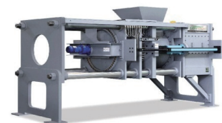
SRF Extruder
